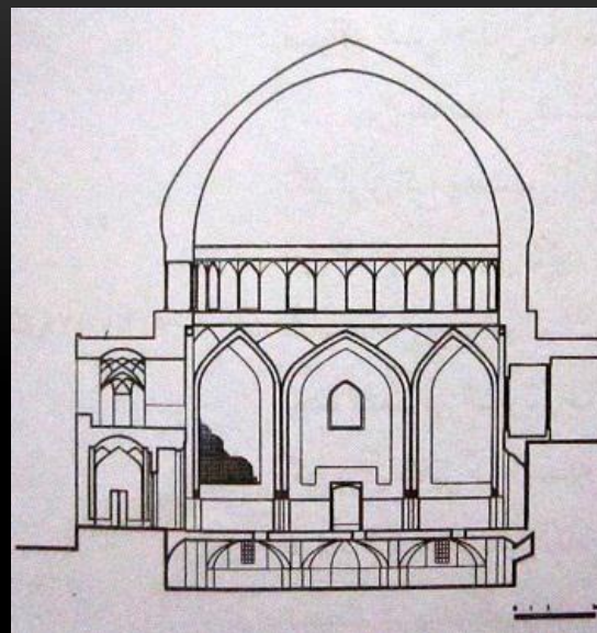
برش
