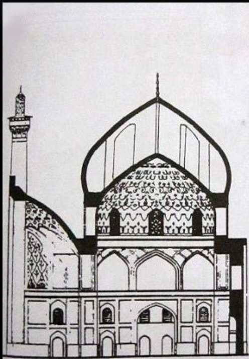
برش گنبدخانه
