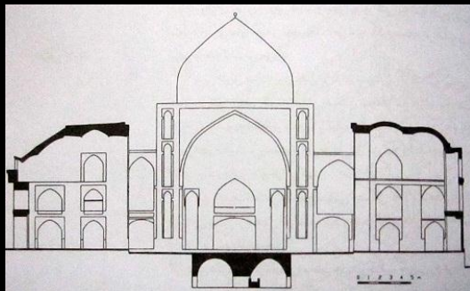
برش عرضی
